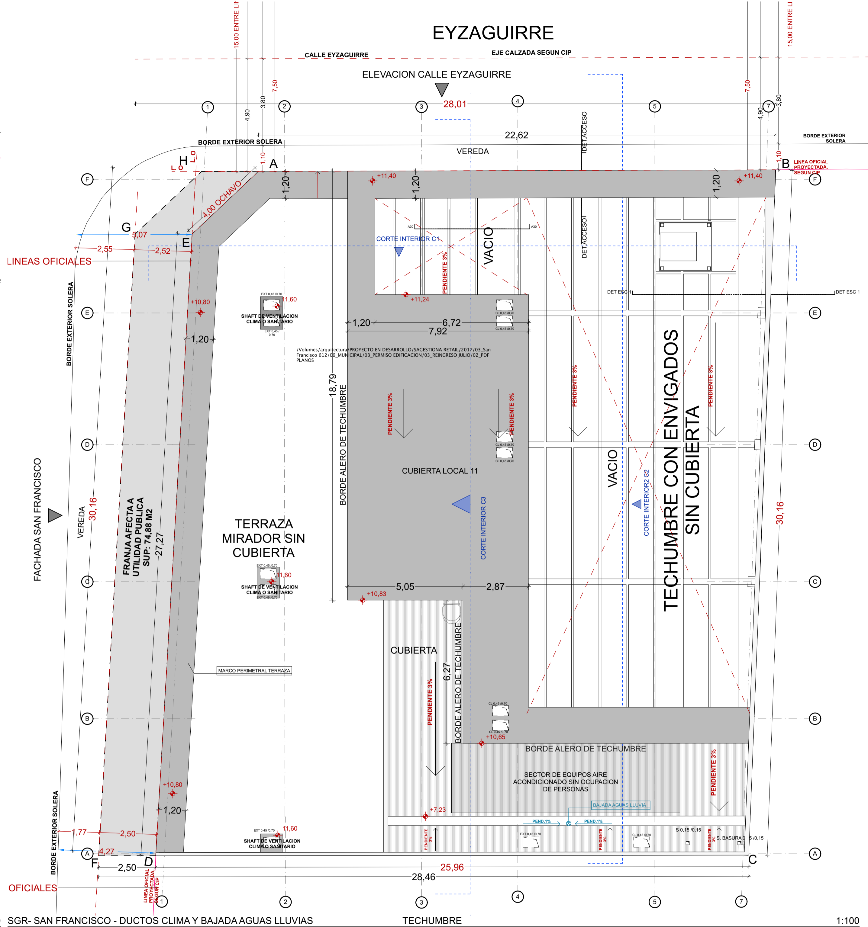
1:100 SGR- SAN FRANCISCO - DUCTOS CLIMA Y BAJADA AGUAS LLUVIAS
