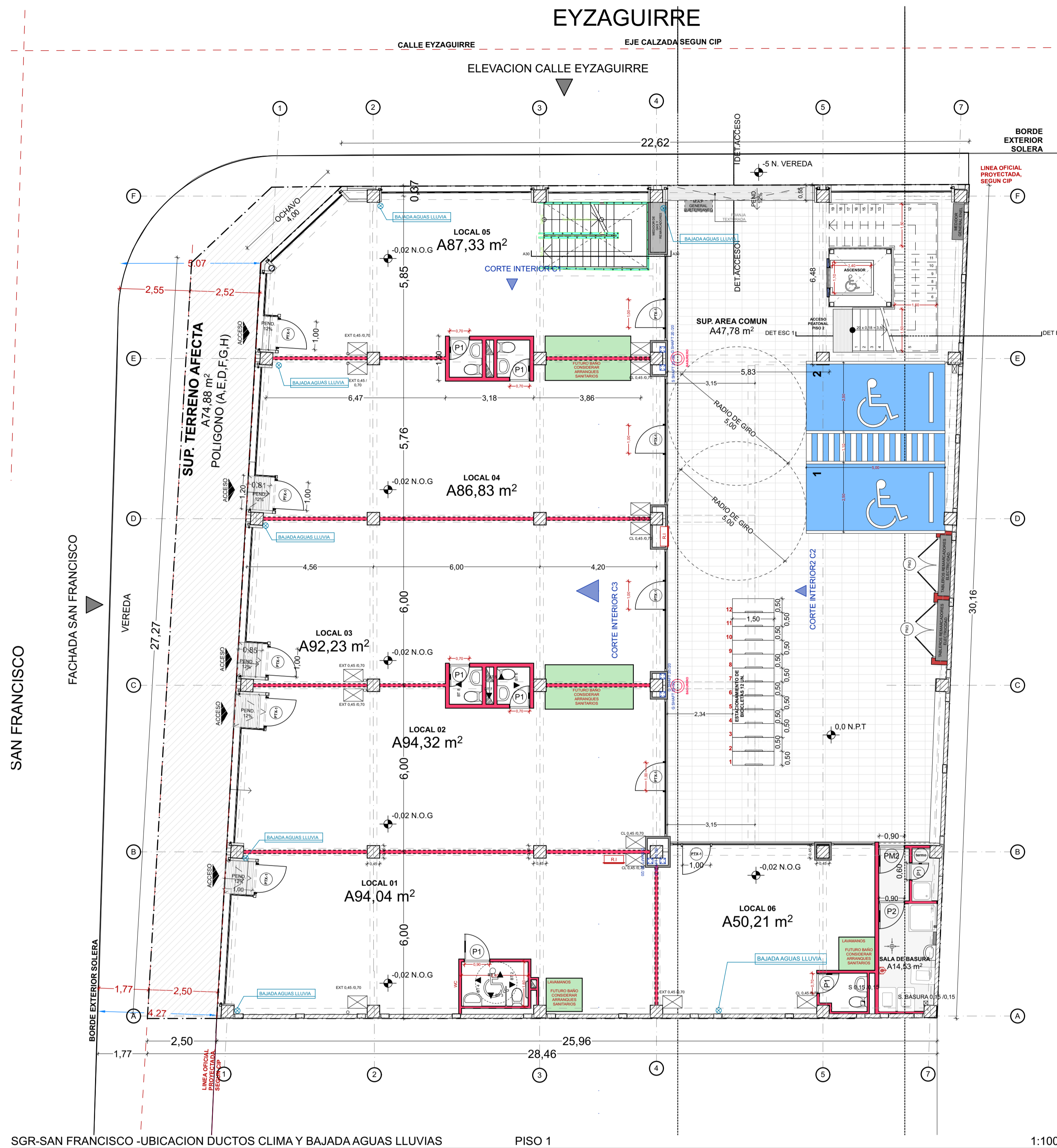
SGR-SAN FRANCISCO -UBICACION DUCTOS CLIMA Y BAJADA AGUAS LLUVIAS
