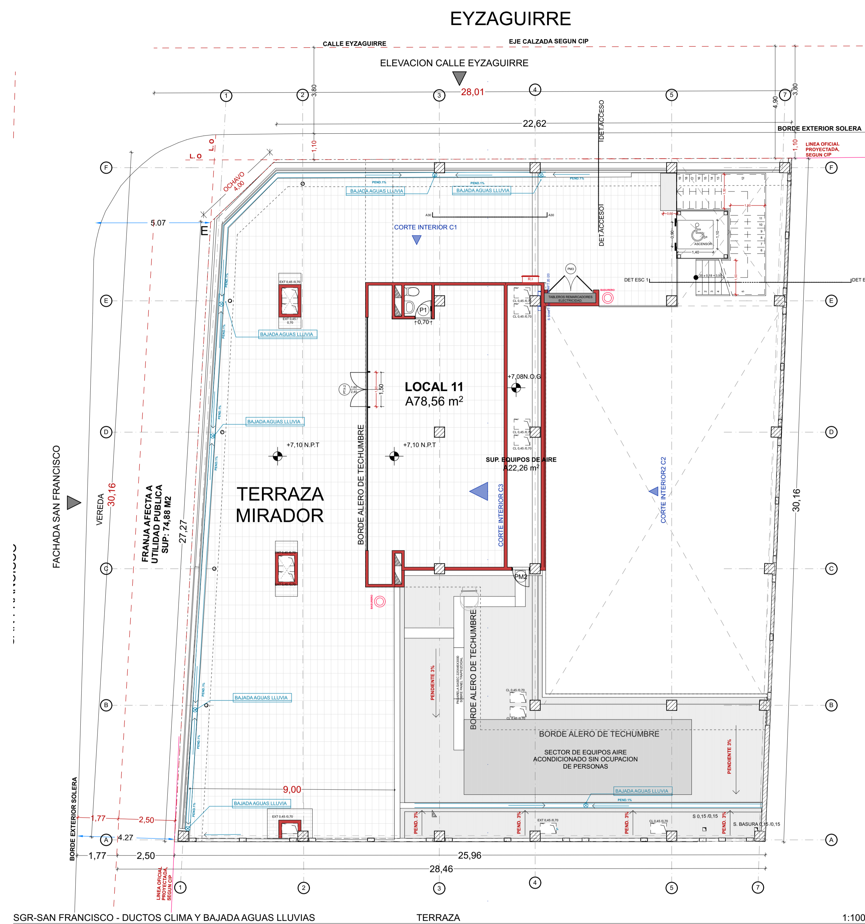
SGR-SAN FRANCISCO - DUCTOS CLIMA Y BAJADA AGUAS LLUVIAS
