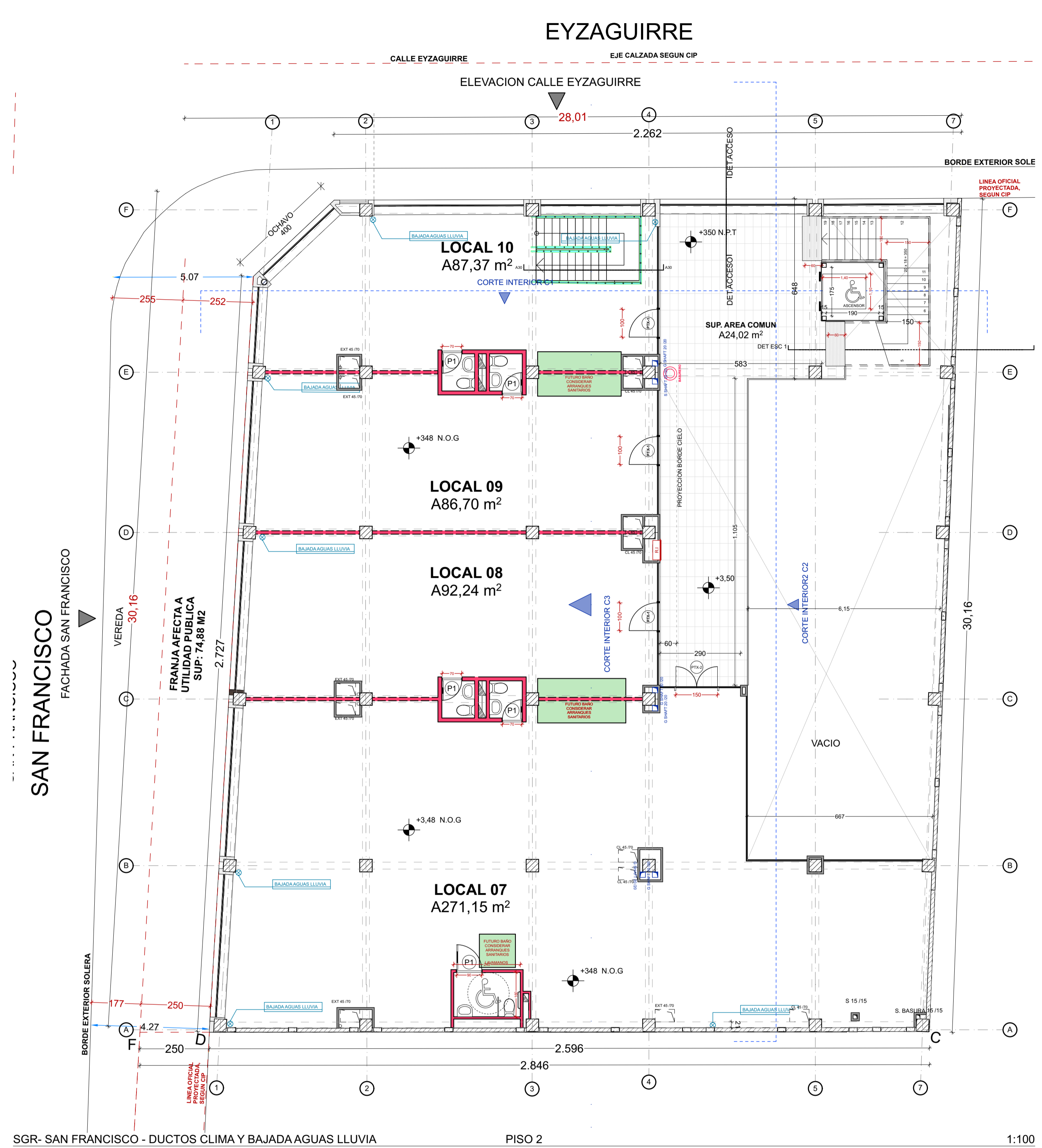
SGR- SAN FRANCISCO - DUCTOS CLIMA Y BAJADA AGUAS LLUVIA
