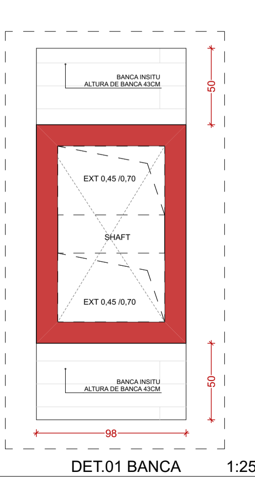
DET.01 BANCA 1:25
